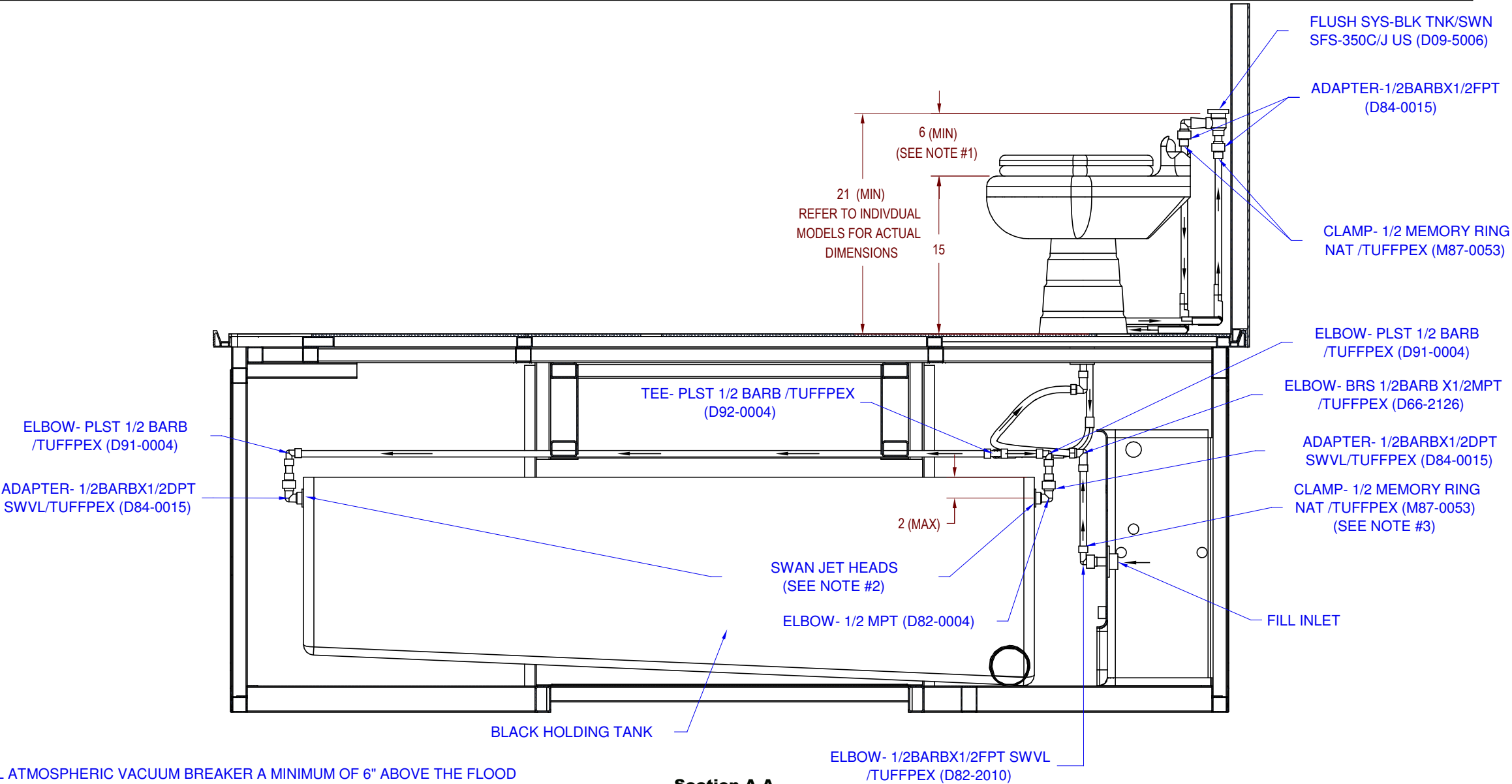
Section A-A
